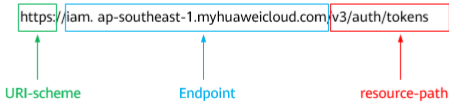
图 2-1 URI 示意图
